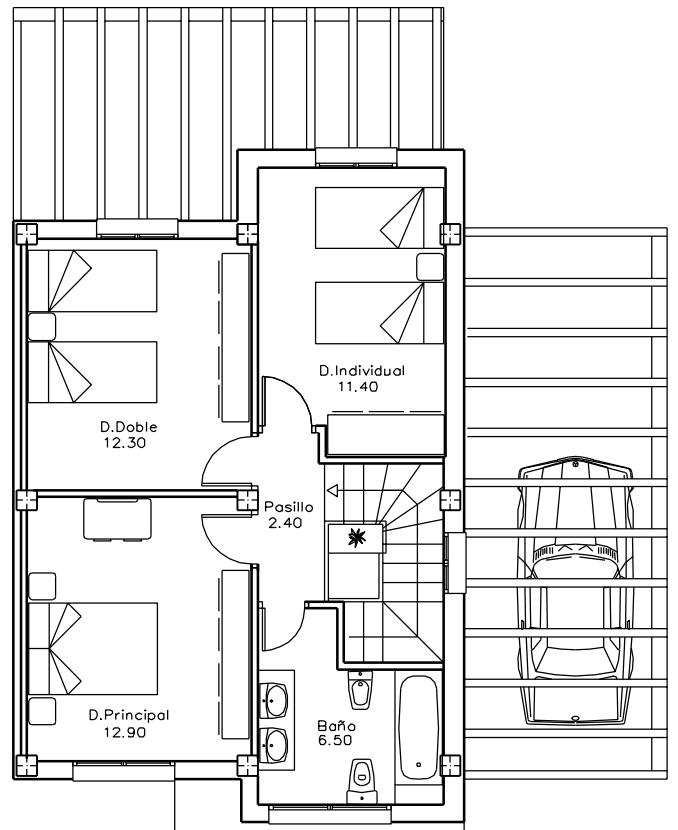
PLANTA PRIMERA 57.00
