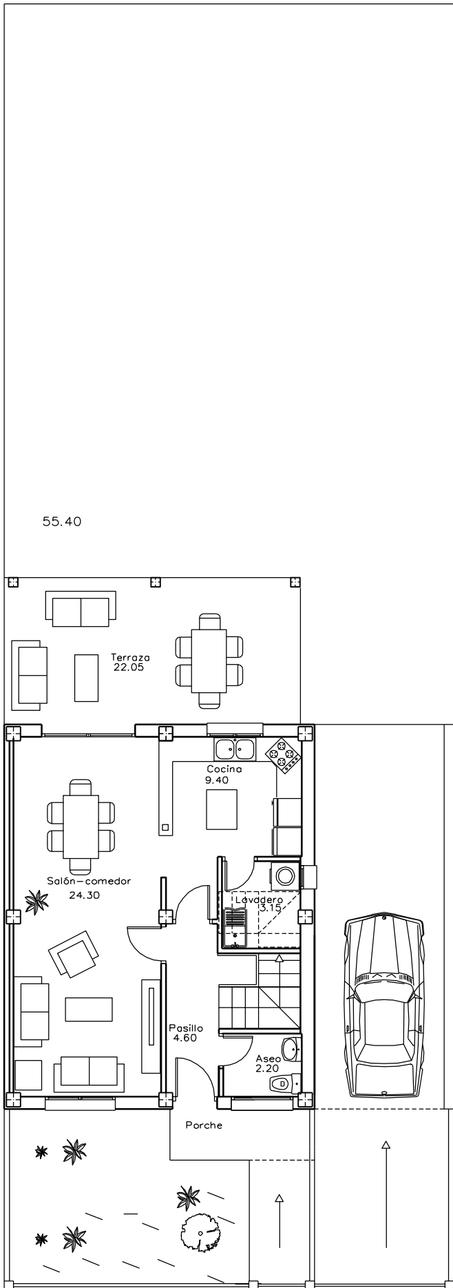
PLANTA BAJA 54.95
