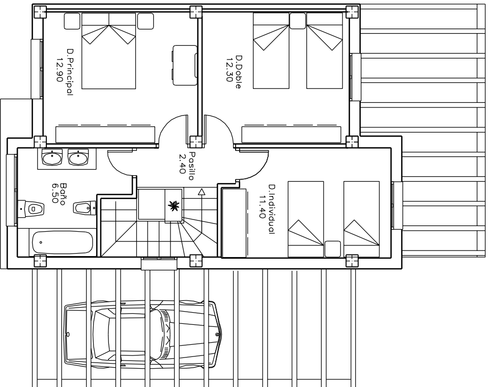
PLANTA PRIMERA 57.00
